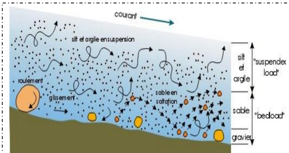
Document 12 : Modes de transports des particules
