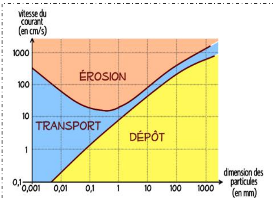
Document 13 : Diagramme de Hjulstrom
