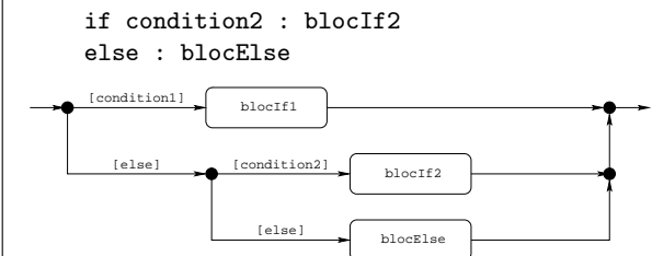
Fig. 2.12 : « if ... else » IMBRIQUÉS if condition1 : blocIf1 else :
